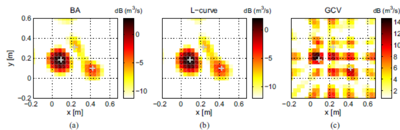
Figure 1: Champs acoustiques reconstruits dans le plan source pour différentes méthodes de régularisation: a) Bayésienne, b) L-curve et c) GCV [5].
